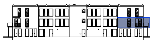
POHLED ZÁPADNÍ
